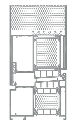
řez PD SP 800 i+
