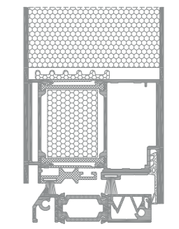
řez PD SP 800 i+
